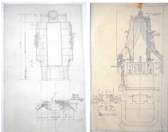
Bitenčevi načrti za oltar božjega groba (dražja in cenejša različica) cerkev sv. Vida, vir: Vinko Žnidaršič
